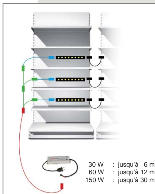
Alimentation électrique optimale de l'éclairage d'étagères avec le système POS 7.
