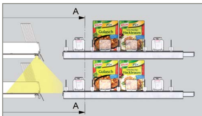
Alimentation électrique optimale de l'éclairage d'étagères avec le système POS 7.
