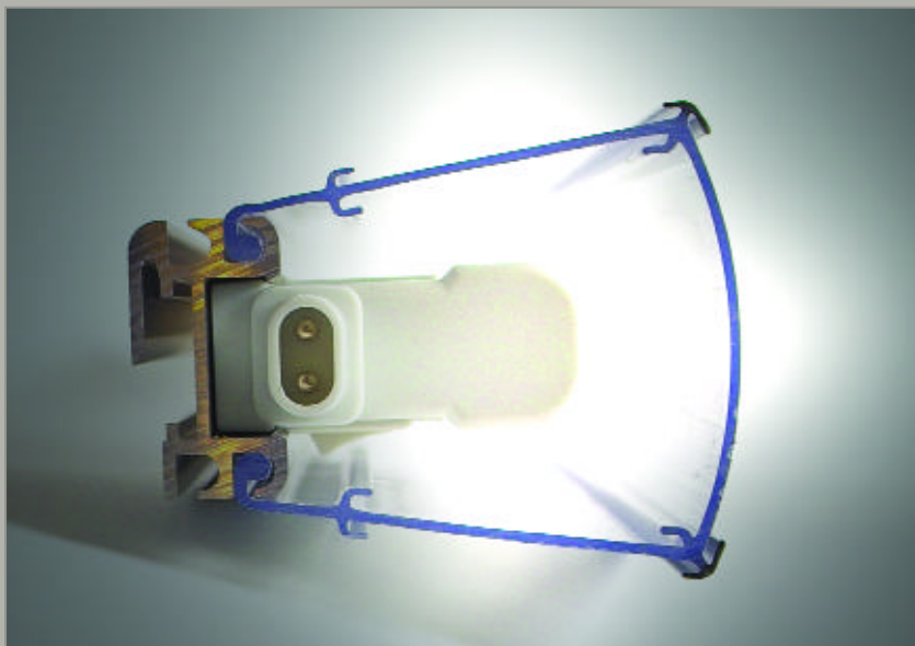
Nuten an Ober- und Unterseite des Chassis bieten zusätzlich die Möglichkeit zur Aufnahme von Scannerschienen.
