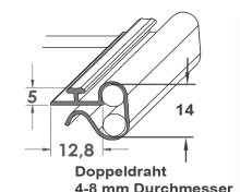
Rail adaptateur T 13, clip pour fil double
