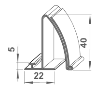
Rail adaptateur T 08, avec bande d'information 40mm, adhésif
