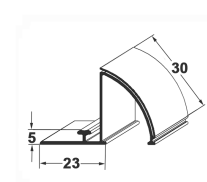
Rail adaptateur T 14, avec bande d'information 30mm, adhésif
