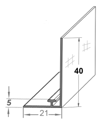
Rail adaptateur T 07, L21mm, rebord 40mm, adhésif
