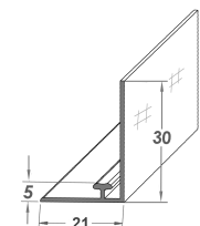
Rail adaptateur T 06, L21mm, rebord 30mm, adhésif
