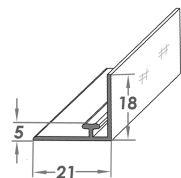
Rail adaptateur T 05, L21mm, rebord 18mm, adhésif
