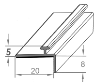
Rail adaptateur T 04, L21mm, m plié 8mm, magnétique
