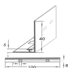
Rail adaptateur T 11, L21mm, rebord 40mm, p. étagères en fil
