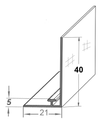
Rail adaptateur T 07, L21mm, rebord 40mm, magnétique
