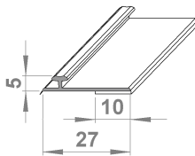
Rail adaptateur T 03, L27mm, avec bande double-adhésive
