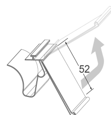
Rail Adaptateur-T 16, avec rail scanner rail pour KIND
