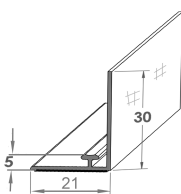
Rail adaptateur T 06, L21mm, rebord 30mm, magnétique
