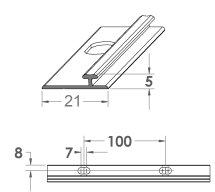
Rail adaptateur T 10, L21mm, p. étagères en fil
