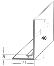
Adapter-T-Profil 07, B21 mm, Aufk. 40 mm, mit Magnet
