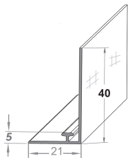
Adapter-T-Profil 07, B21 mm, Aufk. 40 mm, selbstklebend
