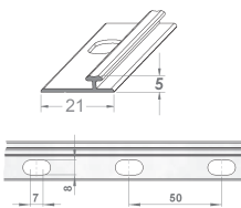
Adapter-T-Profil 10, B21 mm, für Drahtböden
