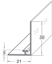
Adapter-T-Profil 06, B21 mm, Aufk. 30 mm, selbstklebend
