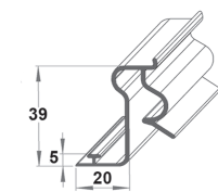
Adapter T-Profil für Drahtböden mit Aufkantung
